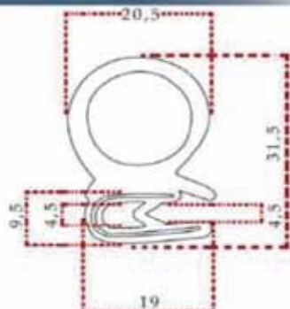
Kapı Ve Bagaj Lastiği Уплотнитель для Дверей и Багажника Doors & Baggage Rubber
