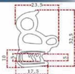
Kapı Ve Bagaj Lastiği Уплотнитель для Дверей и Багажника Doors & Baggage Rubber
