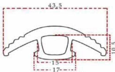
Ray Lastığı Оконный Уплотнитель Vehicles Rail Rubber
