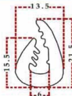
Cam Lastığı Оконный Уплотнитель Vehicles Glass Rubber
