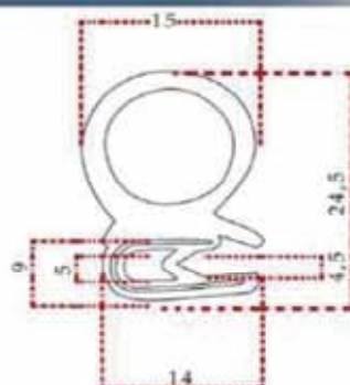
Kapı & Bagaj Lastiği Уплотнитель для Дверей и Багажника Doors & Baggage Rubber
