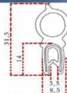
Kapı Ve Bagaj Lastiği Уплотнитель для Дверей и Багажника Doors & Baggage Rubber
