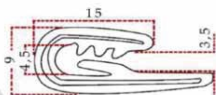
Cam Lastığı Оконный Уплотнитель Vehicles Glass Rubber
