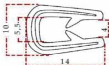
Cam Lastığı Оконный Уплотнитель Vehicles Glass Rubber
